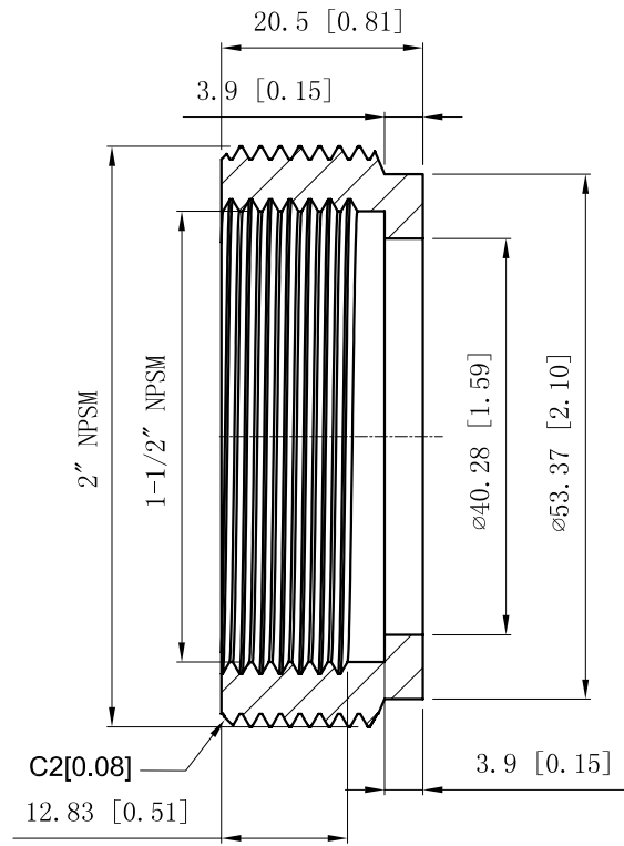
VIEW A-A
