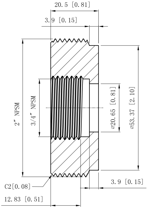
VIEW A-A
